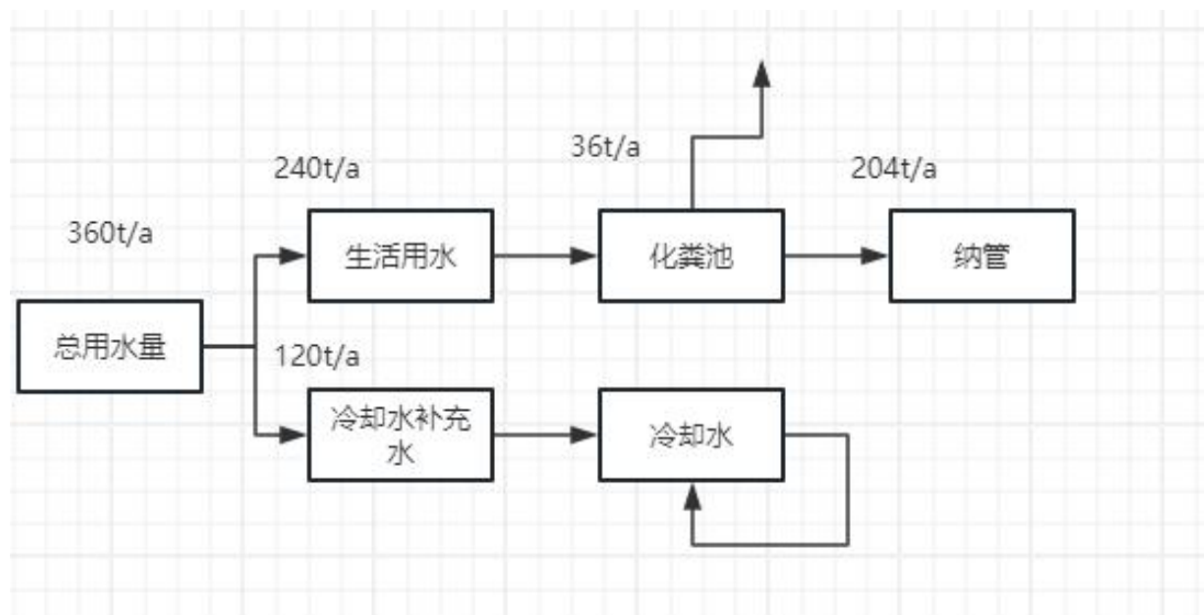
图 2-1 水平衡图
